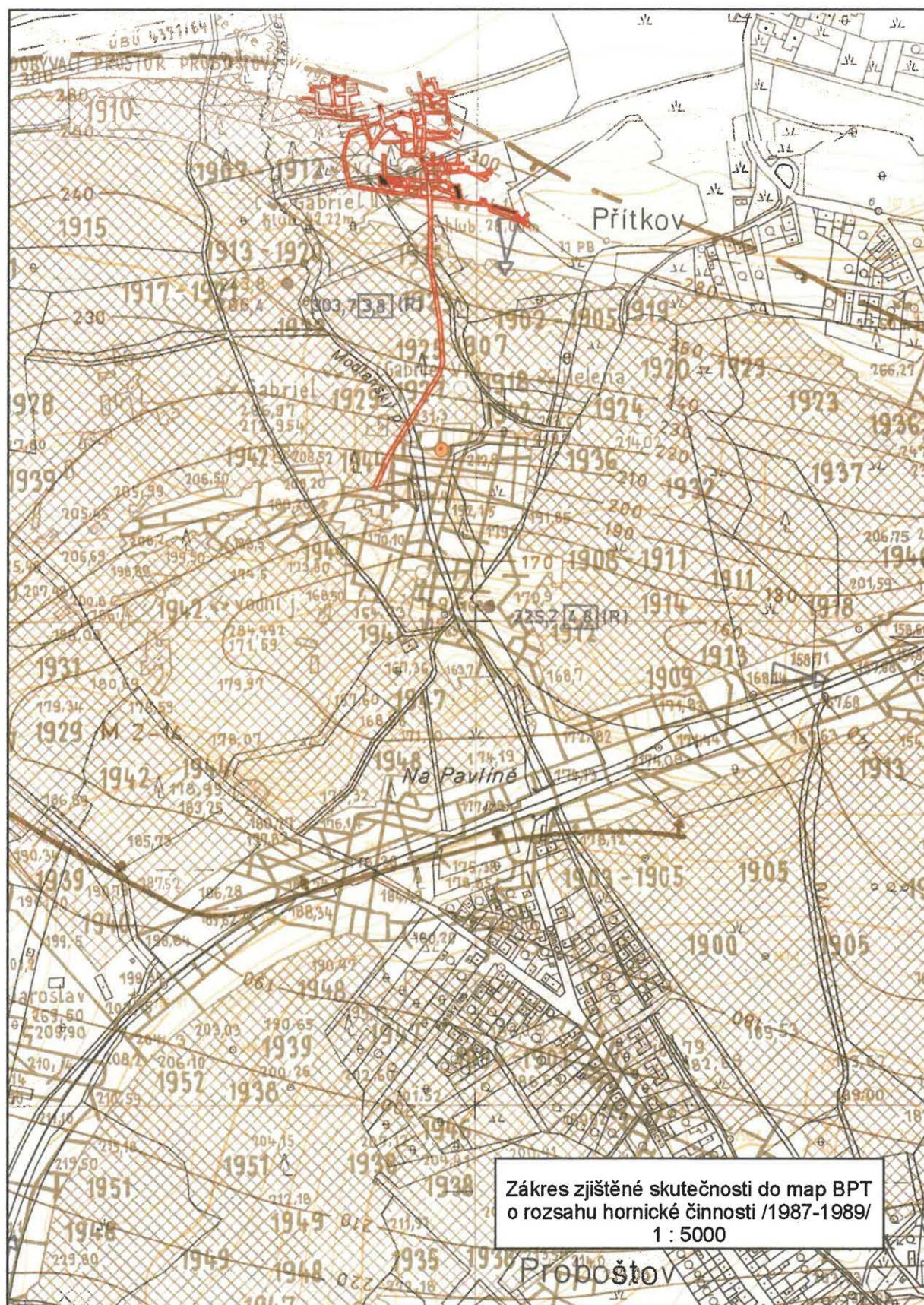
Obr. 3 Zákres zjištěné skutečnosti do map PBT o rozsahu hornické činnosti 1 : 5000, 1987 - 1989
