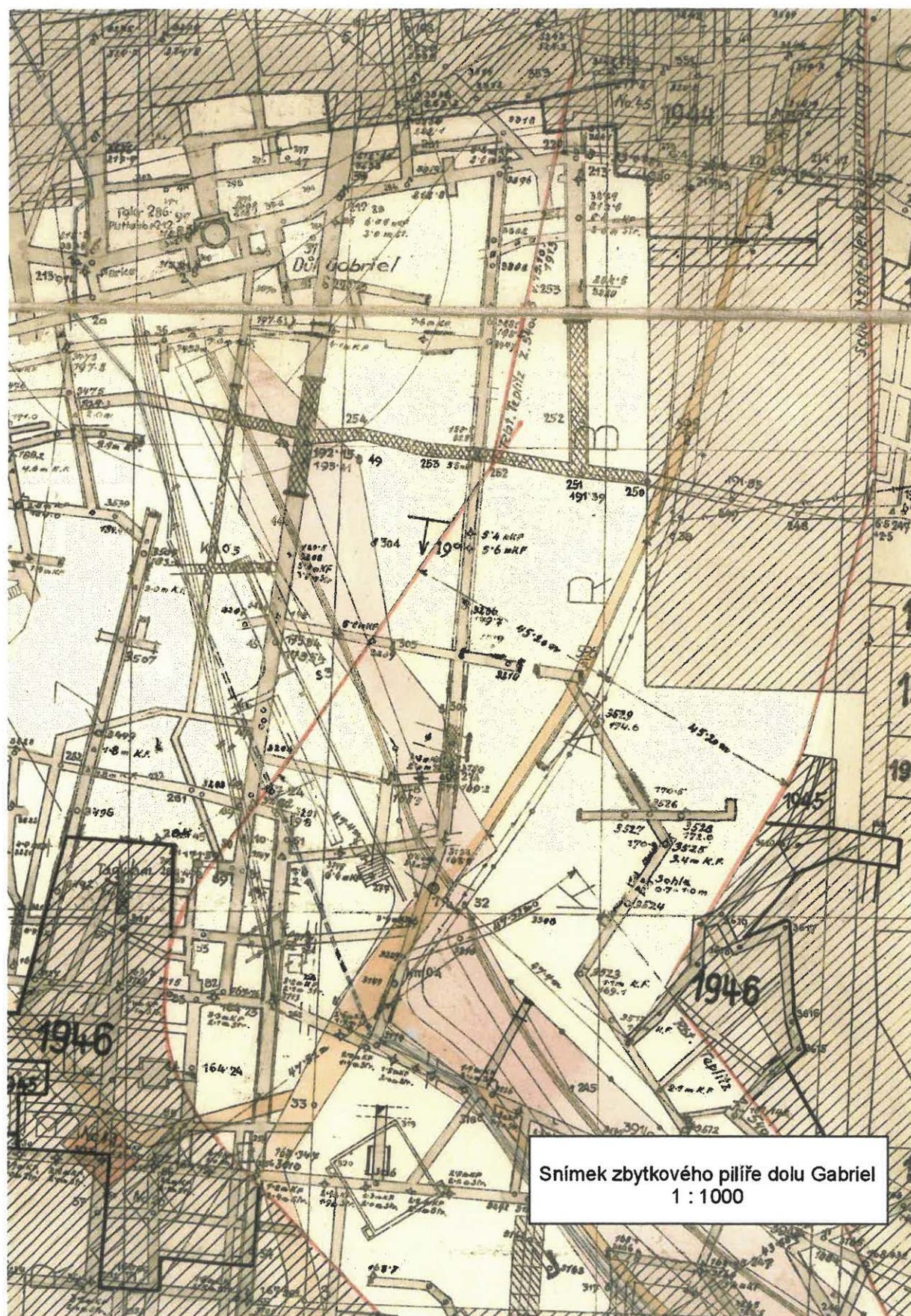
Obr. 2 Snímek zbytkového pilíře dolu Gabriel 1 : 1000
